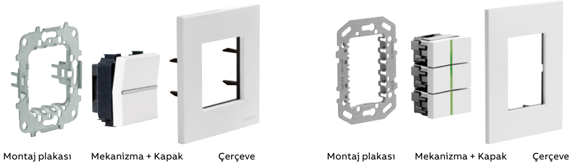
Montaj plakası
